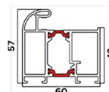
Rysunek techniczny
