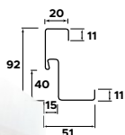
Rysunek techniczny
